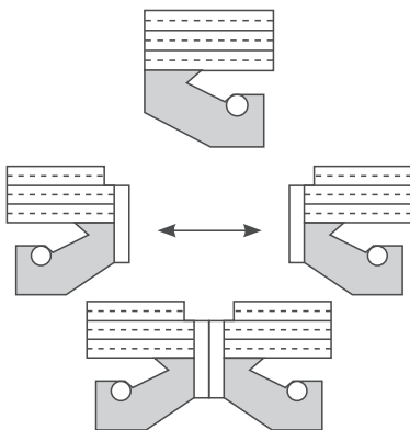
Fig.11 Esempio di montaggio anello tipo FTS Example of installation of FTS seals
