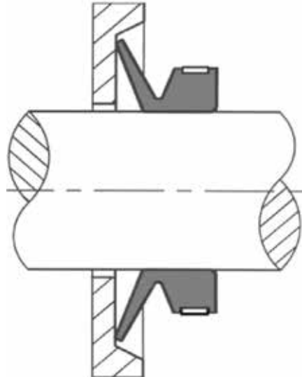
MONTAGGIO TIPO VB CON FASCETTA | TYPE VB INSTALLATION WITH CLAMPING BAND
